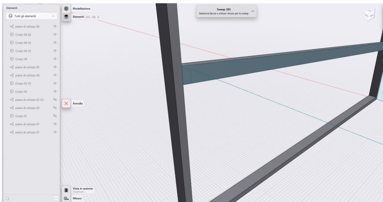
Uso sweep
